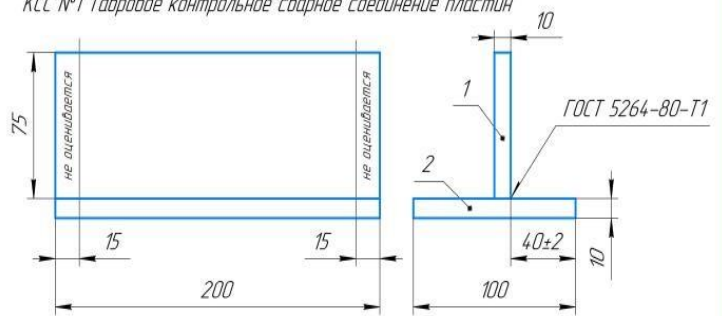
КСС №1 Тавровое контрольное сварное соединение пластин
