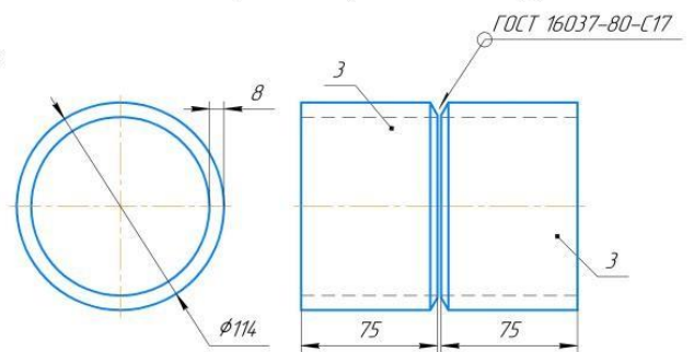
КСС №2 Стыковое контрольное сварное соединение труб
