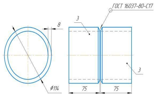
КСС №2 Стыковое контрольное сварное соединение труб
