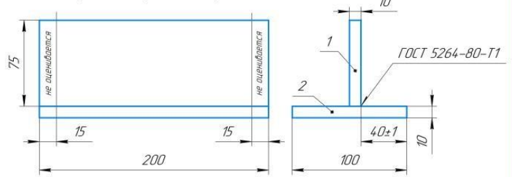
КСС №1 Тавровое контрольное сварное соединение пластин
